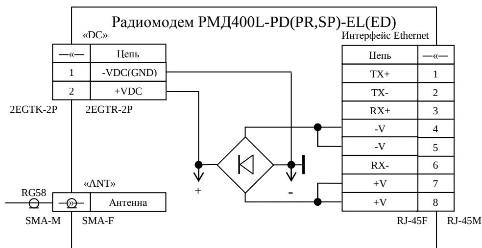
Рис.14 Схема подключения вариантов радиомодема с интерфейсом Ethernet РДМ400L-PD(PR,SP)-EL(ED)
